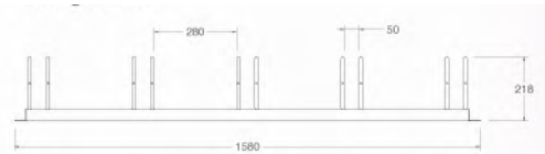
APARCABICIS GALVANIZADO 5 PLAZAS
